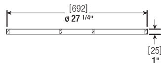
GRILLE DE SÉCURITÉ ACIER GALVANISÉ GS-28-42-G
