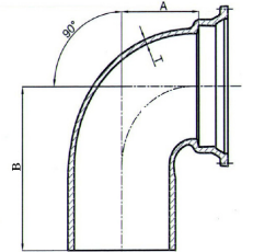
MJ x PE Bend 90°
