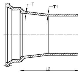
PE x MJ (large end MJ)
