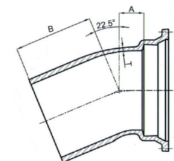
MJ x PE Bend 22-1/2°
