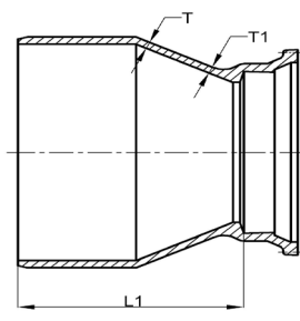
PE x MJ (small end MJ)
